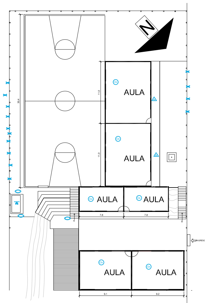
PLANTA ARQUITECTÓNICA
