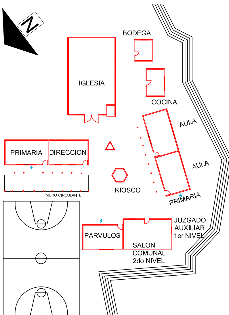
PLANTA ARQUITECTÓNICA
