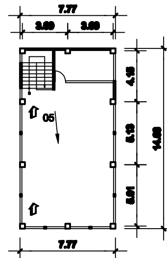
PLANTA NIVEL 4
