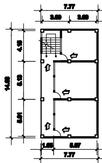
PLANTA NIVEL 2 Y 3
