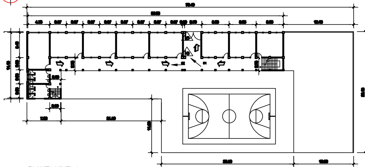
PLANTA NIVEL 1
