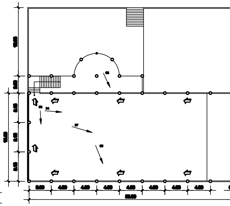
PLANTA NIVEL 2
