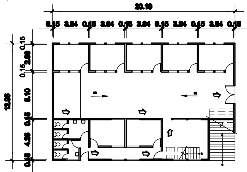
PLANTA NIVEL 1
