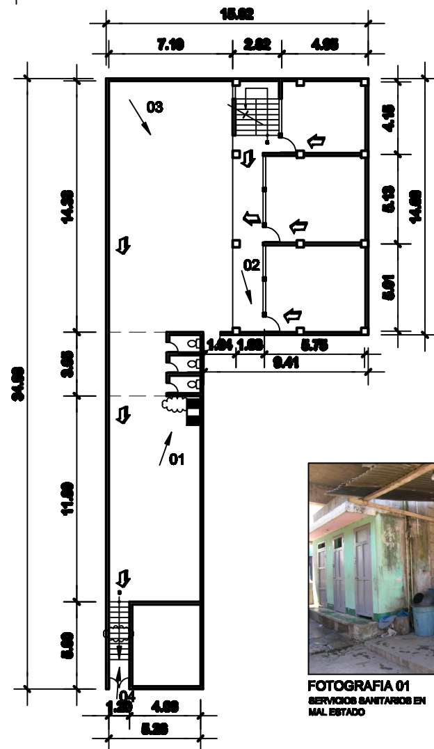
PLANTA NIVEL 1
